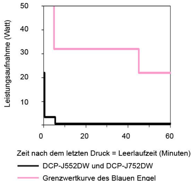
Leistungsaufnahme und Aktivierungszeiten des DCP-J552DW und DCP-J752DW in der Zeit nach dem letzten Druck
