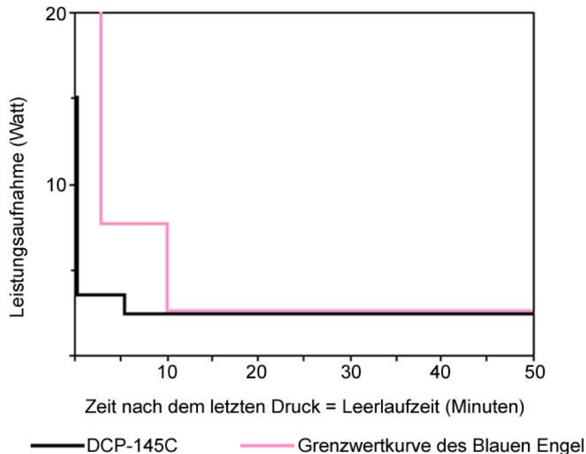
Leistungsaufnahme und Aktivierungszeiten des DCP-145C in der Zeit nach dem letzten Druck
